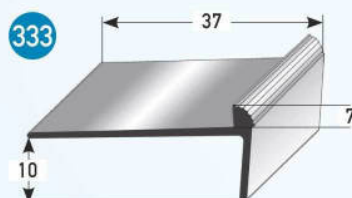
Schodová hrana 10x37x7mm z hliníku
