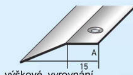
výškové vyrovnání
