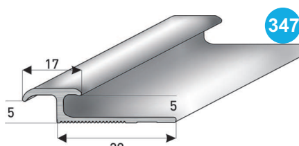
dvojitý zásuvný profil 5mm
