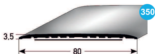
přechodový profil 80x3,5mm
