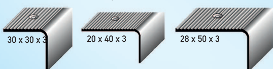
Nerezová ocel, 3mm, frézovaná
