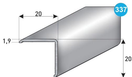
OCHRANA ROHŮ - 20x20mm
