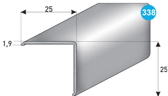
OCHRANA ROHŮ - 25x25mm
