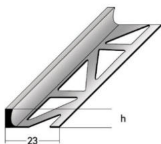
Profil pro dlažbu oddělovací profil
