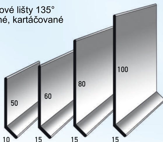
Ochrana rohů Délka 1,0 ; 1,25; 2,5m
