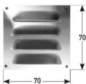
Lüftungsblech/ vents
