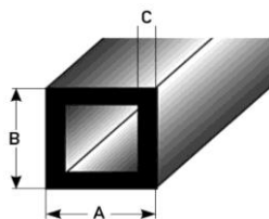
Čtyřhranný profil
